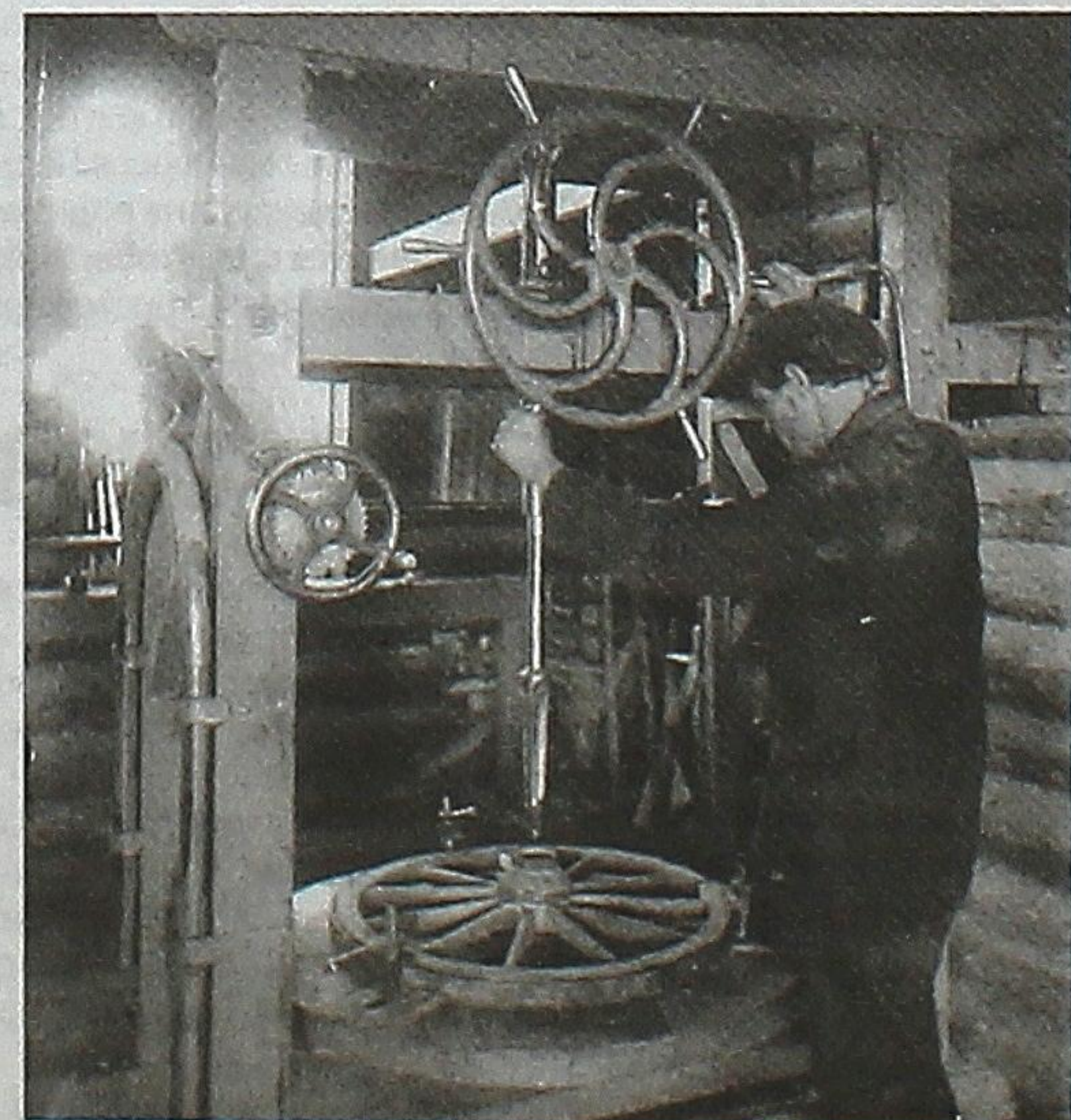
Вертикально-сверлильный станок для овтуливания колес в кустарно-промысловой артели Красный Молот, 1948 г.
